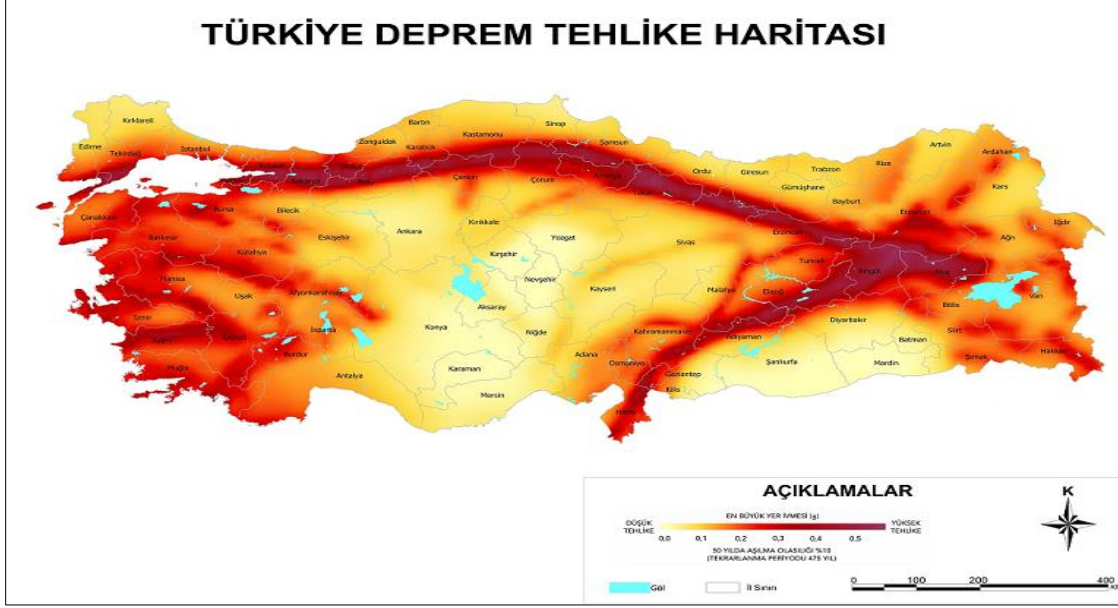
Şekil 6.2: Türkiye Deprem Tehlike Haritası
