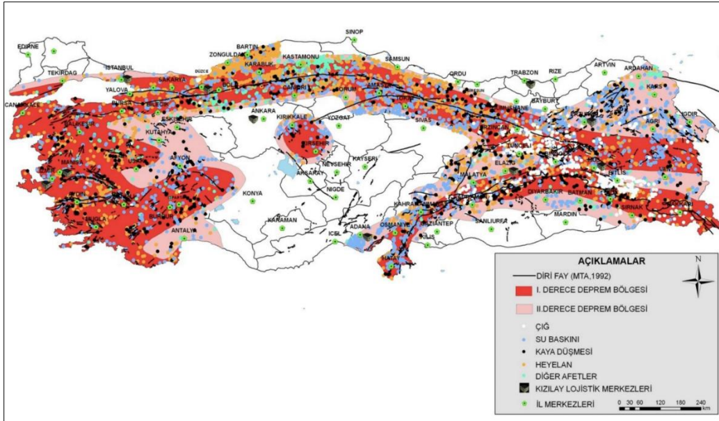
Şekil 6.1: Türkiye Afet Haritası
